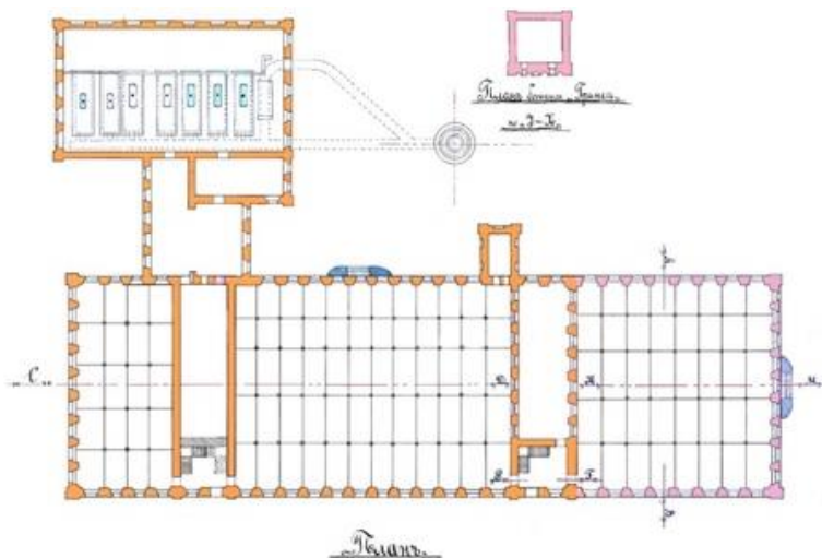
Рис. 1. План прядильного корпуса. Проект пристройки справа (выделена розовым цветом стен) и надстройки гринельной башни. Архивный чертеж 1895 г.
