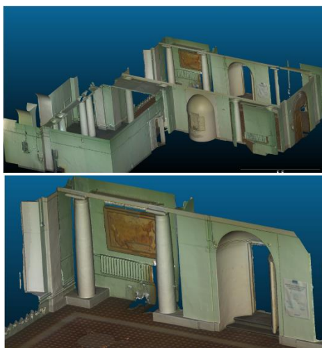
Рис. 4. Модель интерьера в разрезе
