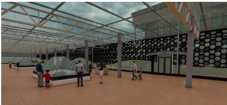
Рис. 4. Проектное предложение по организации на заводе по производству яхт остекленного пространства на крыше с пирамидальными фонарями для осмотра производственного процесса
